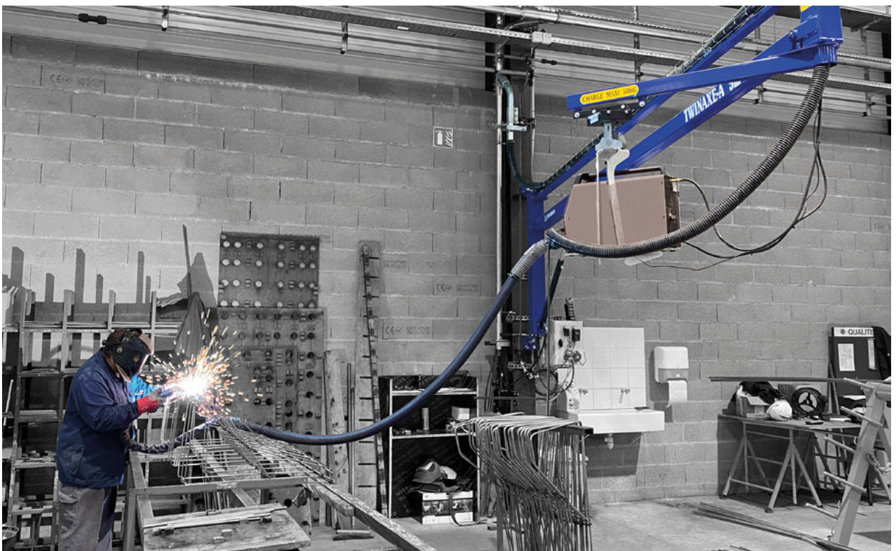
Potence TWINAXE ajustable et torche aspirante
